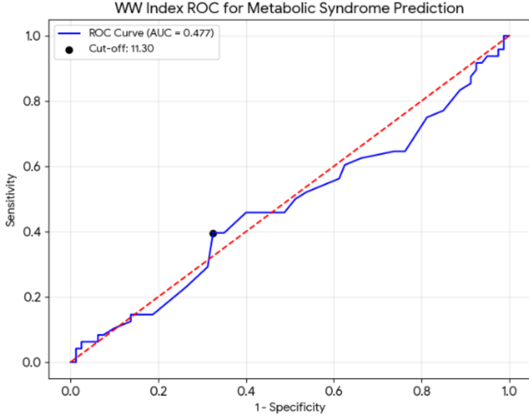
WWI için MS öngörü değerlendirme ROC analizi
