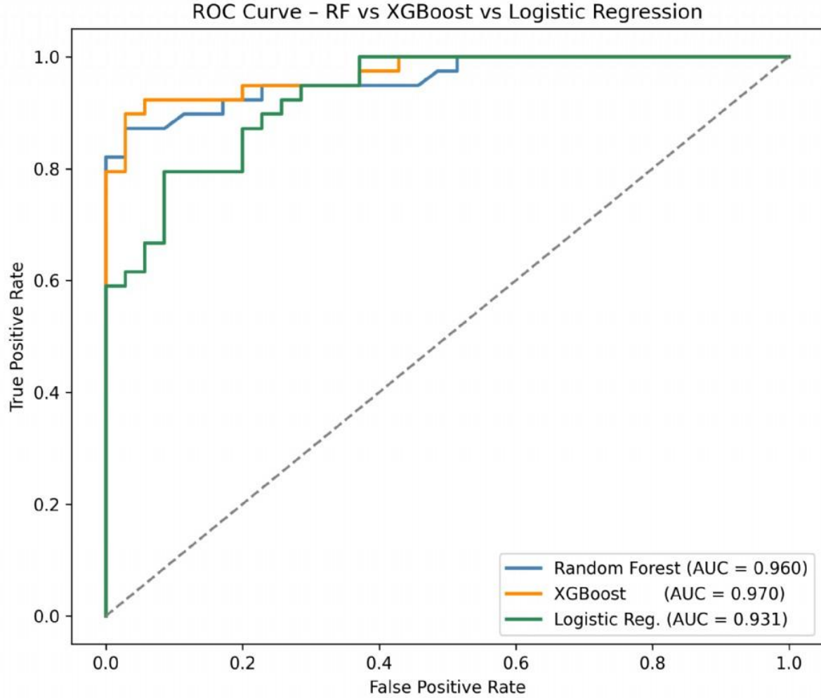
Şekil 2: Rastgele Orman, Aşırı Gradyan Artırma ve Lojistik Regresyon Modellerine Ait ROC Eğrileri ve AUC Değerleri
