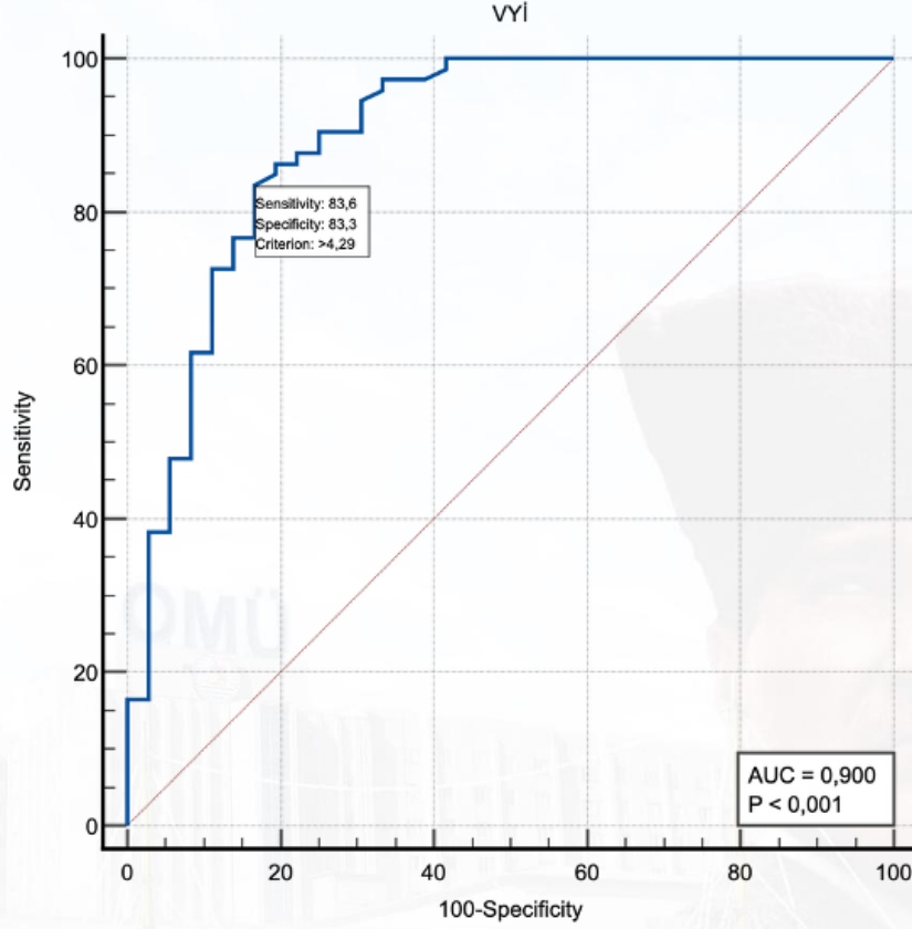
Şekil 1. Vücut Yuvarlaklık İndeksi (VYİ) Ölçümünün Obezite Tanısını Öngörmedeki Performansına Ait ROC Eğrisi
