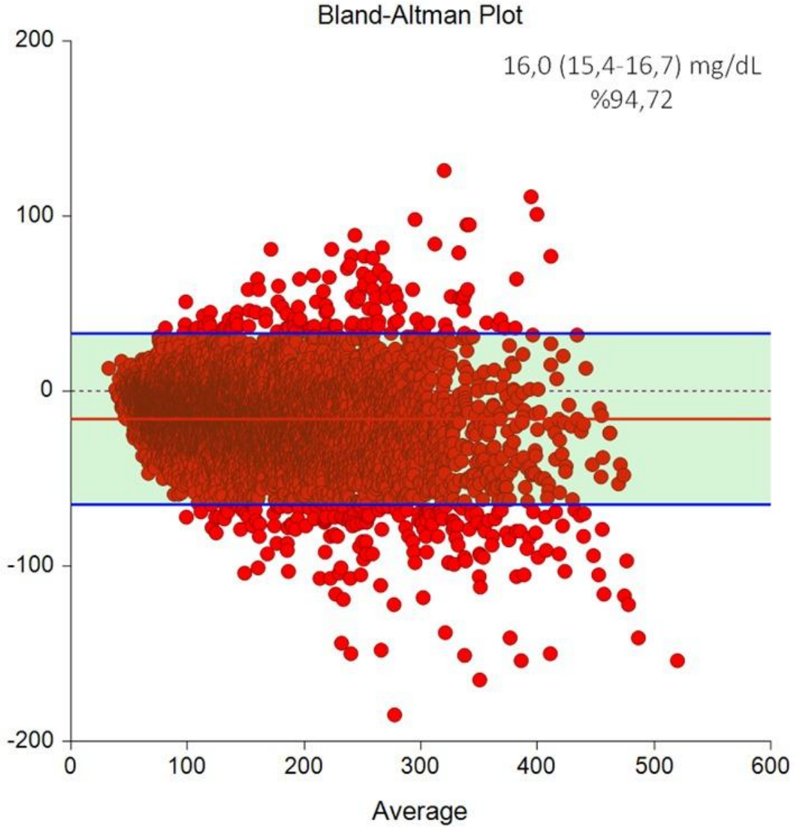
Figür 2: Bland–Altman Grafiği
